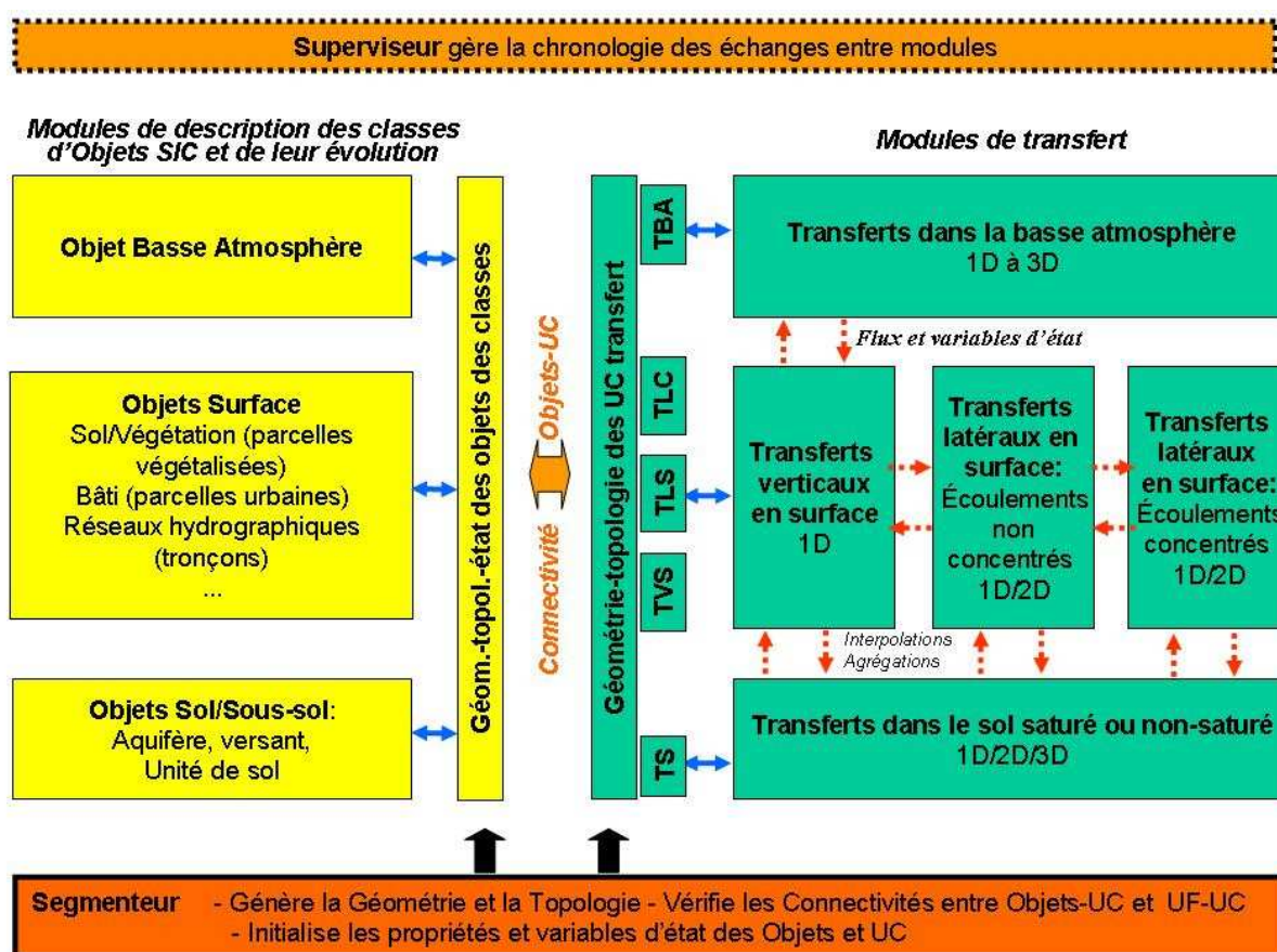
Figure 4. : Schéma de l'architecture du modèle SEVE
